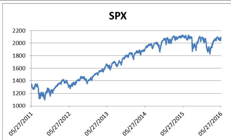
Ovanstående diagram visar kursutvecklingen för S&P 500® Index på S&P Dow Jones Indices LLC..
