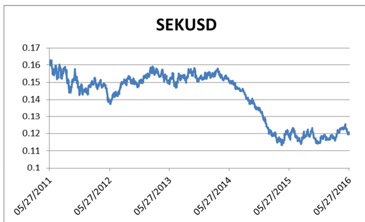
Ovanstående diagram visar kursutvecklingen SEK/USD, det vill säga priset för en svensk krona (SEK) uttryckt i amerikanska dollar (USD). En fallande kurva visar att den SEK försvagats i förhållande till USD. Det krävs färre antal USD för att köpa en SEK
